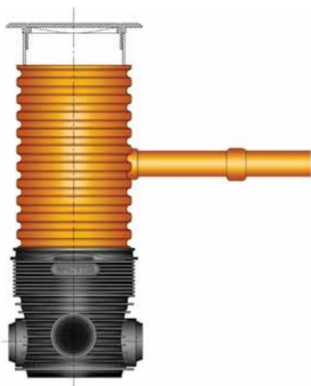
Przykładowe rozwiązania kaskad przy studzienkach niewłazowych
